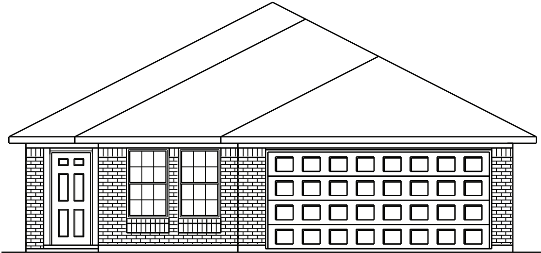
ELEVATION A
